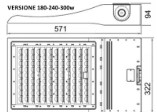
Montaggio TestaPalo
