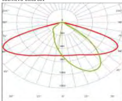
SOLAREVO-ottica 801
