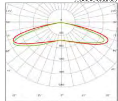
SOLAREVO-ottica 805
