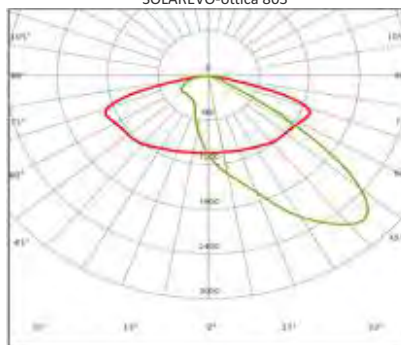
SOLAREVO-ottica 803
